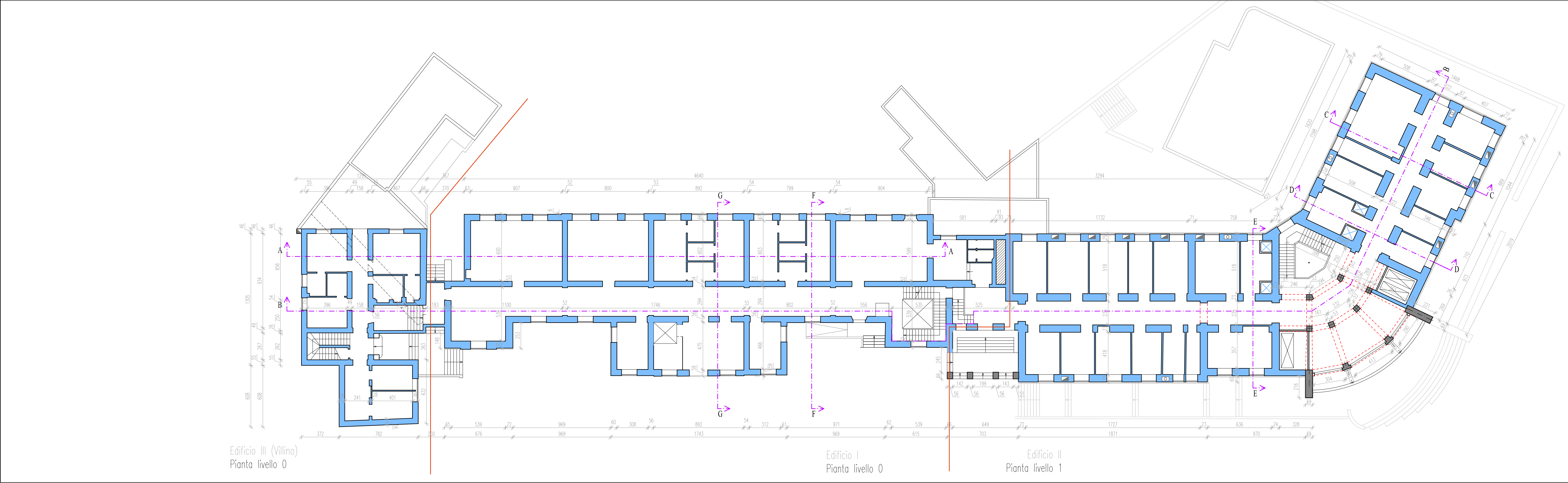
Edificio I Corridoio compreso tra livello -1 e livello 0
